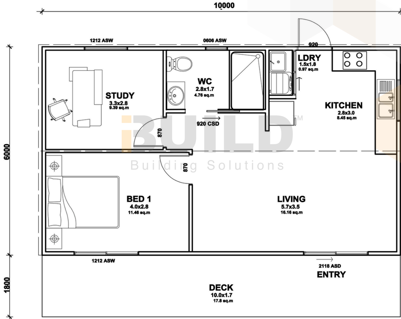
*UPDATED FLOORPLAN 2025.01.23
